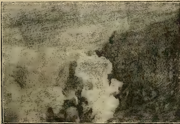
FIG. 3.—VULCANO. THE CRATER.
